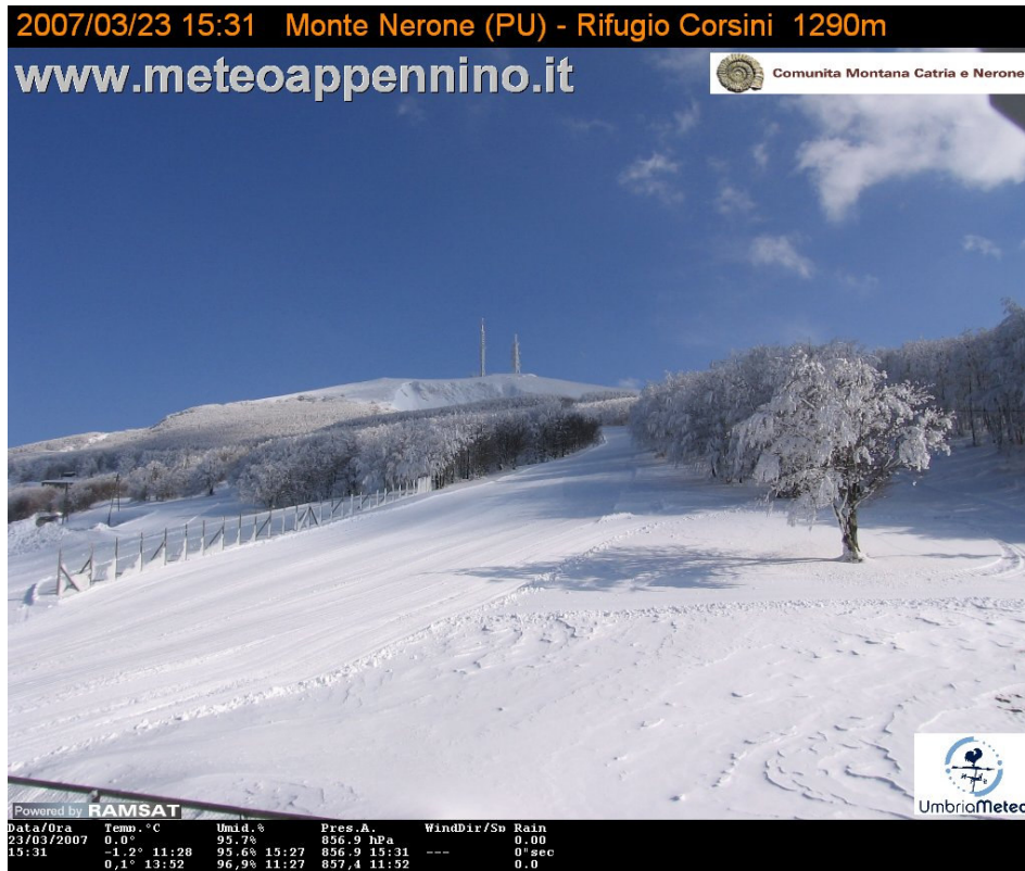
SITO DI INSTALLAZIONE Rifugio Corsini – Monte Nerone: sistema webcam integrato con sensore meteo
